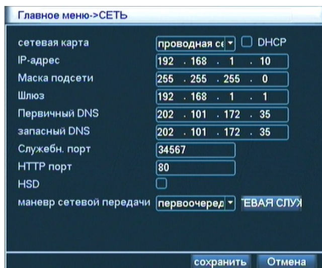
Рис. 4.4 Настройка сети
